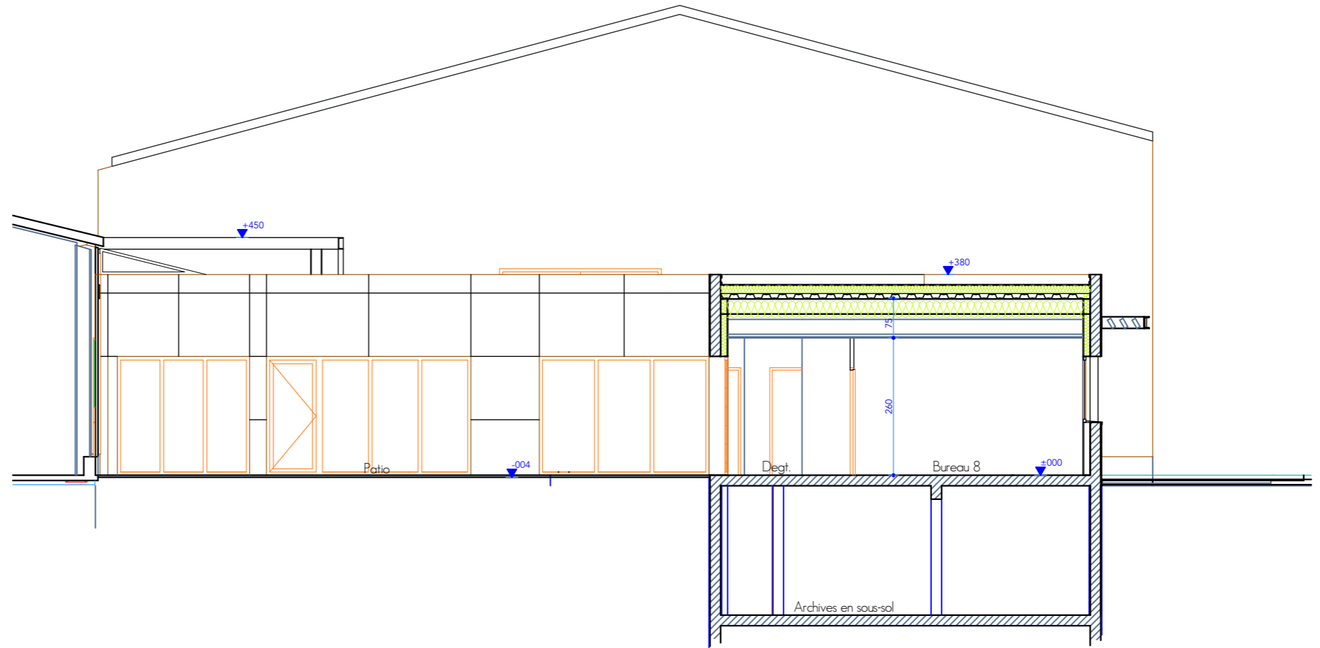
Coupe sur Patio
